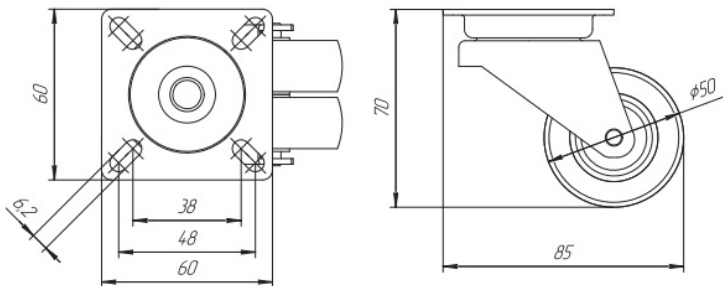
Рис.1 - Чертеж поворотных роликов.
